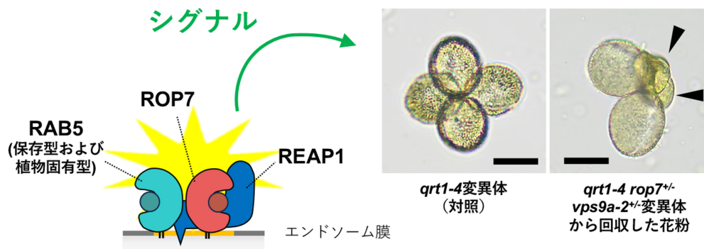
図4： RAB5-REAP1-ROP7 分子ネットワークは正常な花粉形成を支える： RAB5、REAP1、ROP7 がはたらく分子ネットワークの模式図（左）。対照（ qrt1-4 変異体）と比較し、ROP7 と RAB5 の活性が同時に低下した変異体（ qrt1-4 rop7 -/- vps9a-2 -/- 変異体）では、約半分の花粉四分子に異常な花粉（矢尻）が観察された（右）。VPS9A は RAB5 の活性化因子で、 vps9a-2 変異体では RAB5 の活性が低下している。スケールバーは 20 \mu\text{m} 。
